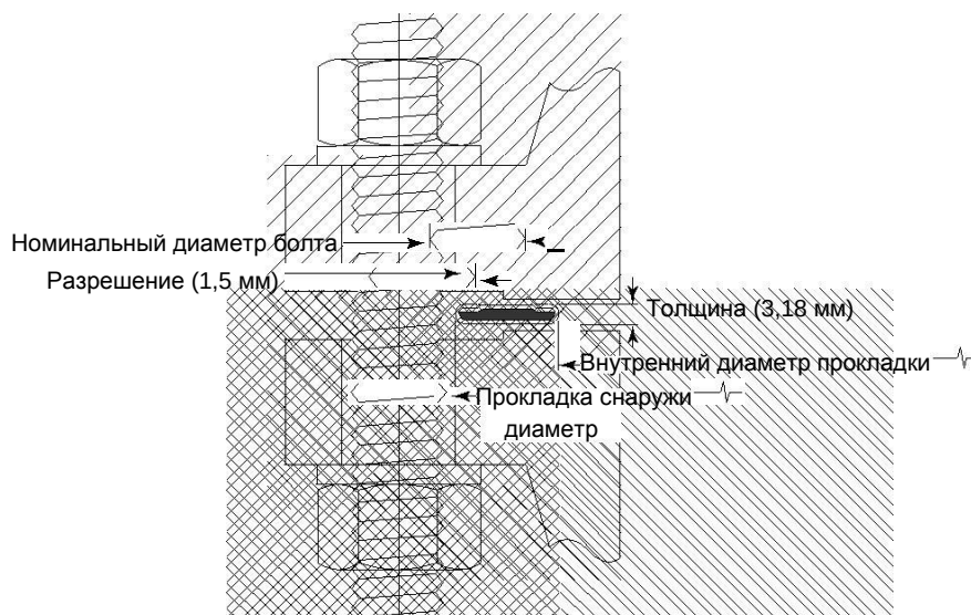
Рис. 2 Покрытые кожей прокладки (метрика)
