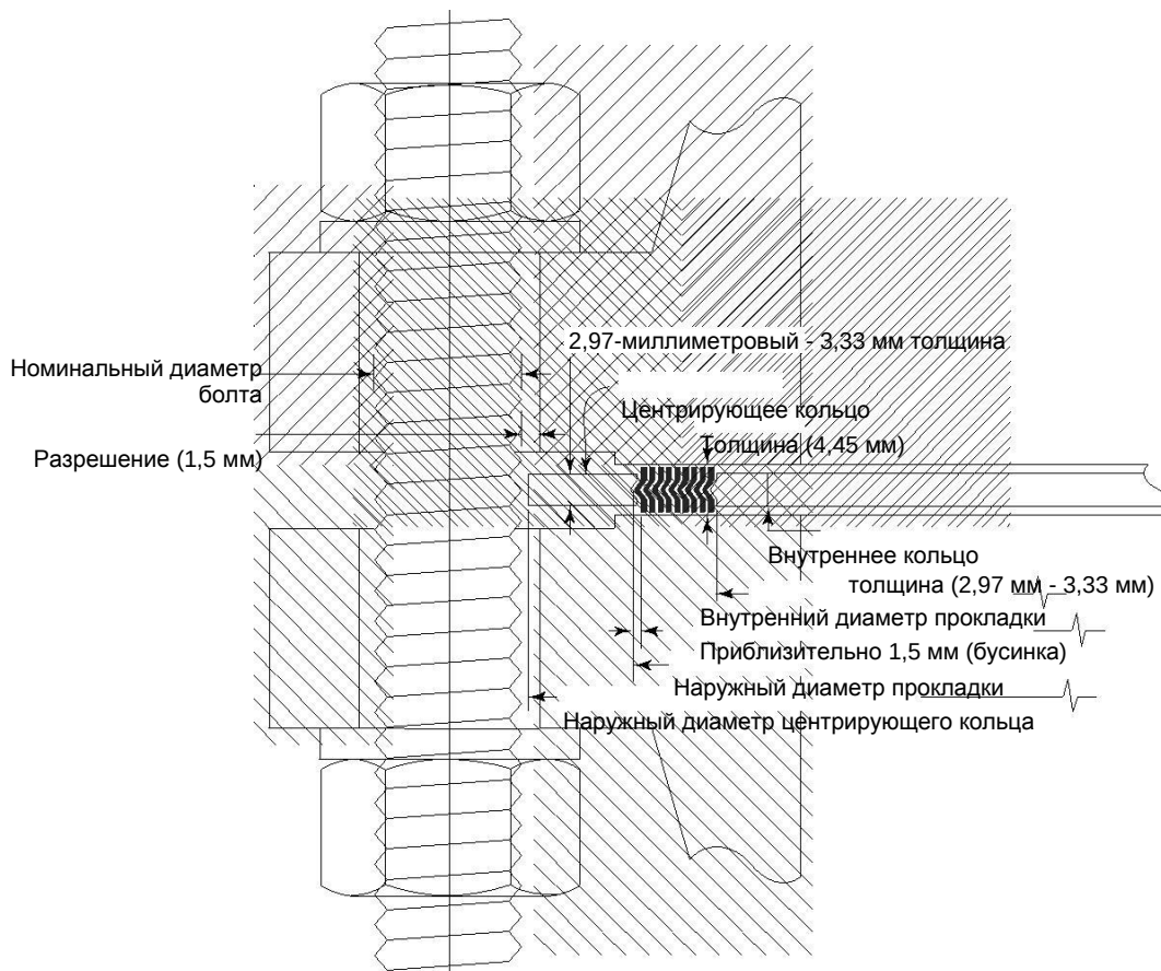
Рис. 1 Прокладки из проволоочных спиралей (метрика)
