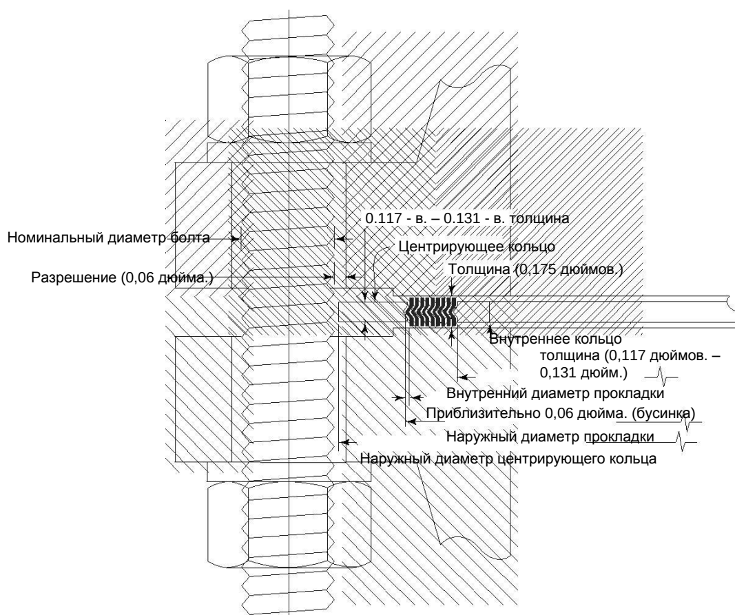
Рис. i-1 Прокладки из проволоочных спиралей (США. Обычный)
