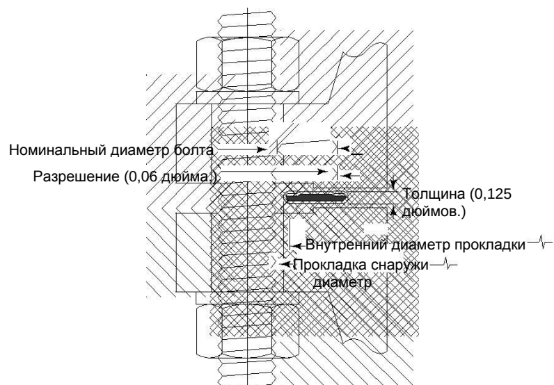
Рис. i-2 Покрытые кожухом прокладки
